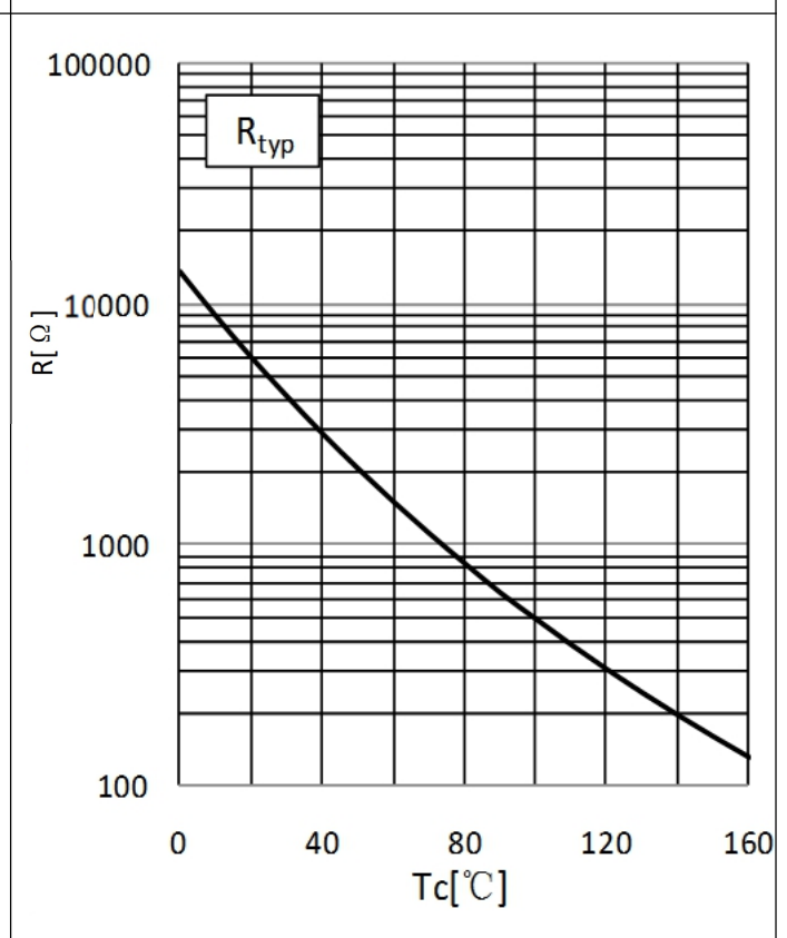
Fig.12:Typ. NTC-Temperature Characteristics 图 12: 典型的 NTC 电阻-温度特性
