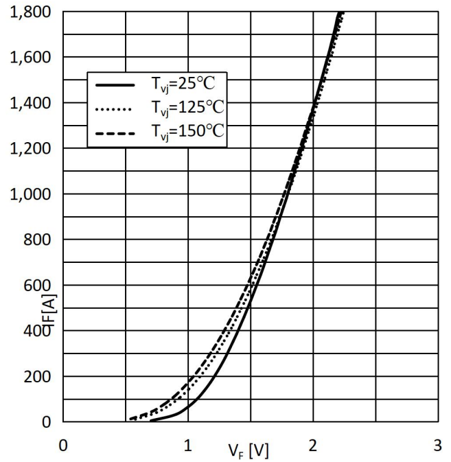
Fig.8: Forward characteristic 图 8: 正向特性
