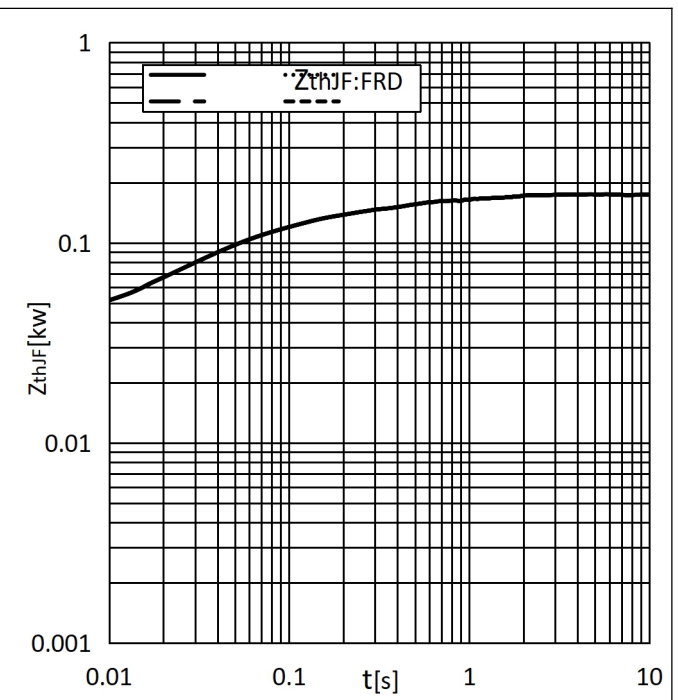
Fig. 14: Typ. transient thermal impedance(FRD) Z_{thJF} FRD(K/W)
