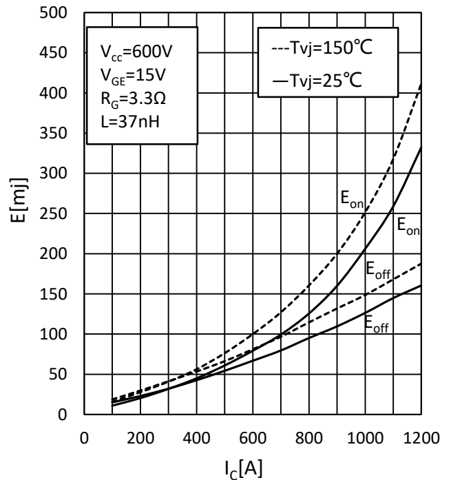
图 4 开关损耗和集电极电流
