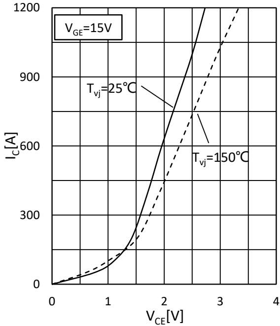
图 1 开通状态特性
