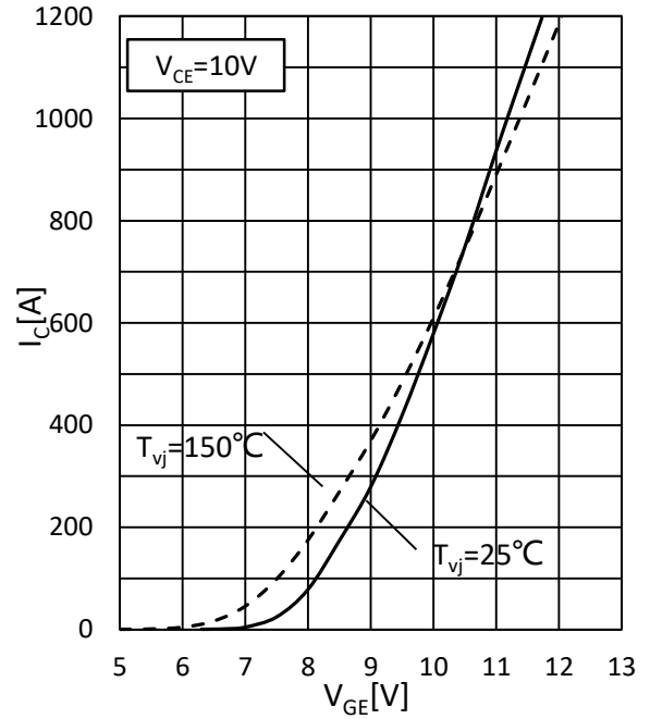
图 2 传输特性
