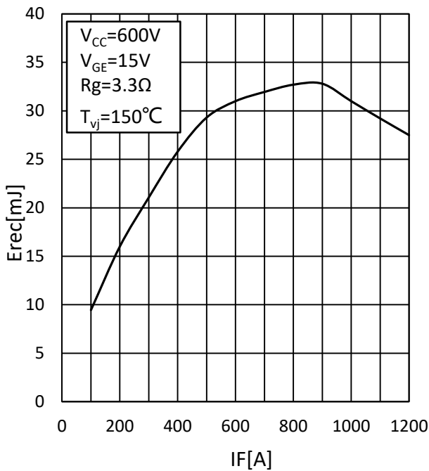
图 7 开关损耗二极管-逆变器
