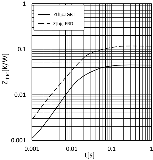
图 9 瞬态热阻
