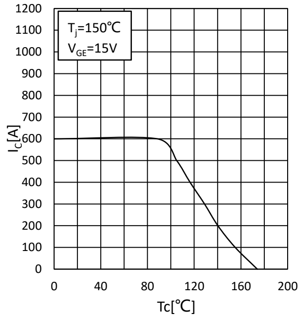
图 10 额定电流和温度
