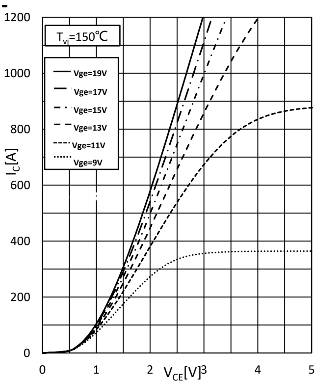
图 3 输出特性
