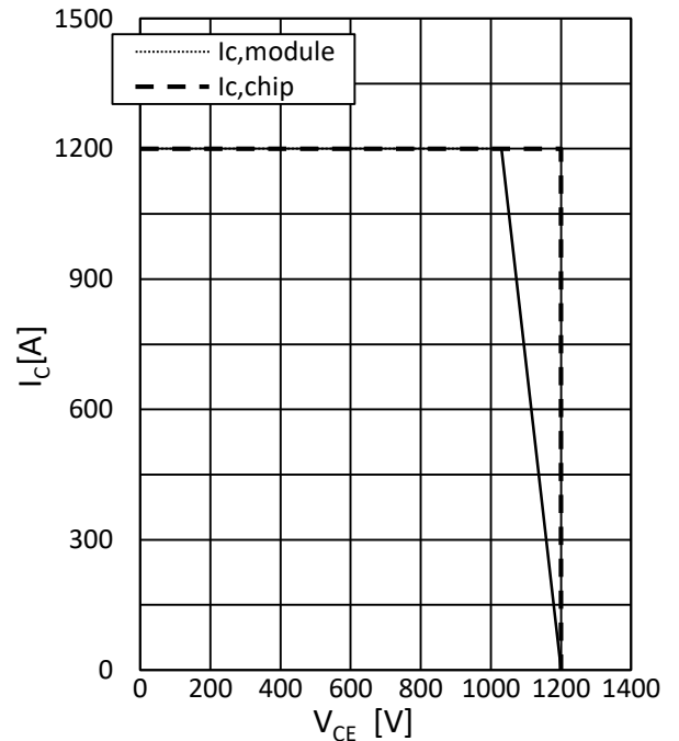
图 8 反偏安全工作区
