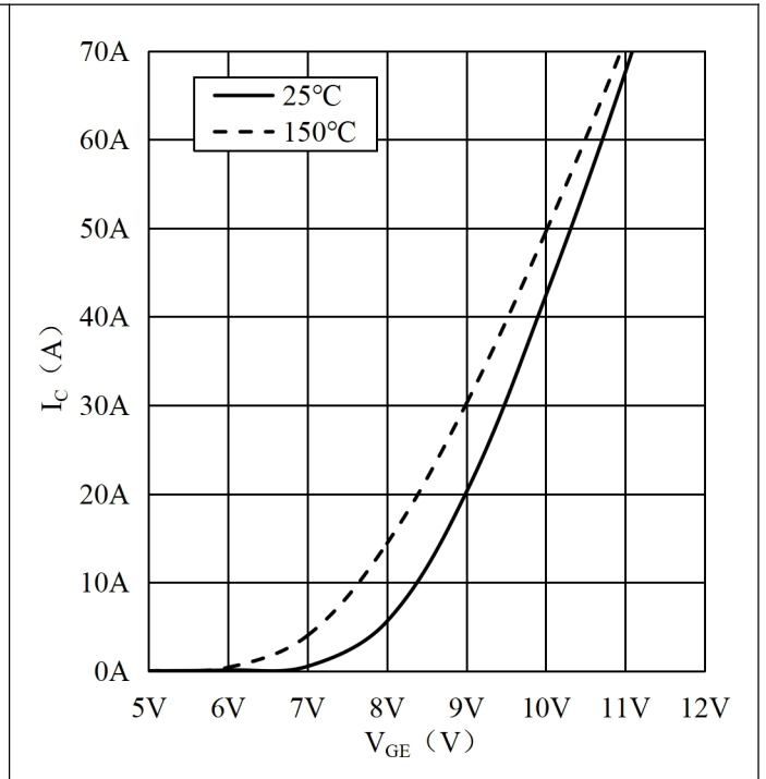
Fig.2 Typ. Transfer Characteristics-Inverter 图 2 传输特性-逆变器
