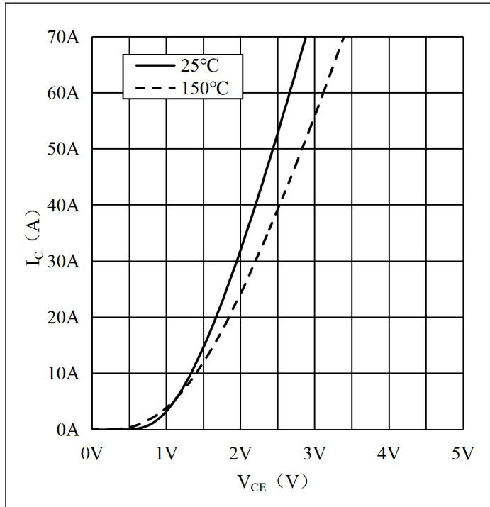
Fig.1 Typ. Output Characteristics-Inverter 图 1 输出特性-逆变器
