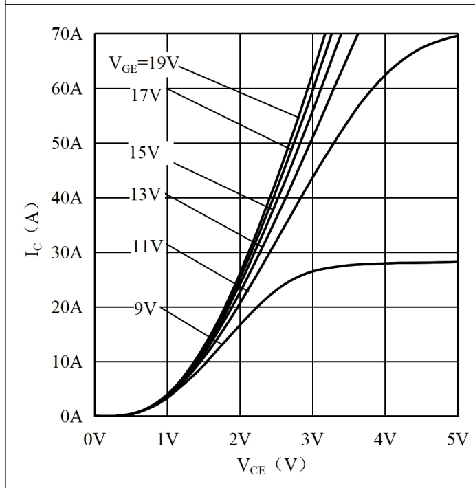
Fig.3 Typ. Output Characteristics-Inverter 图 3 输出特性-逆变器
